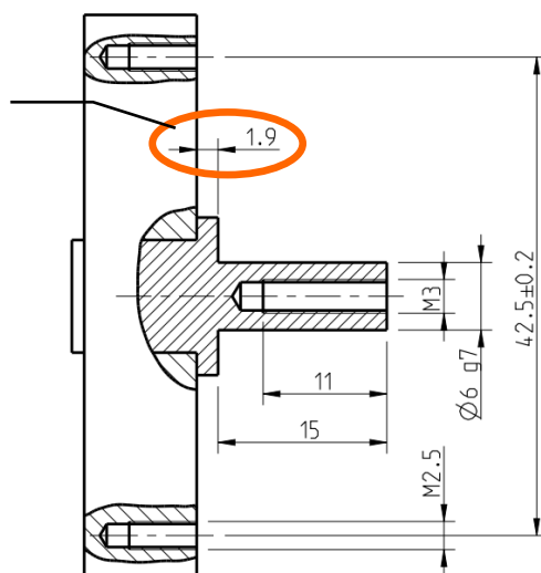
编码器安装推荐尺寸要求
